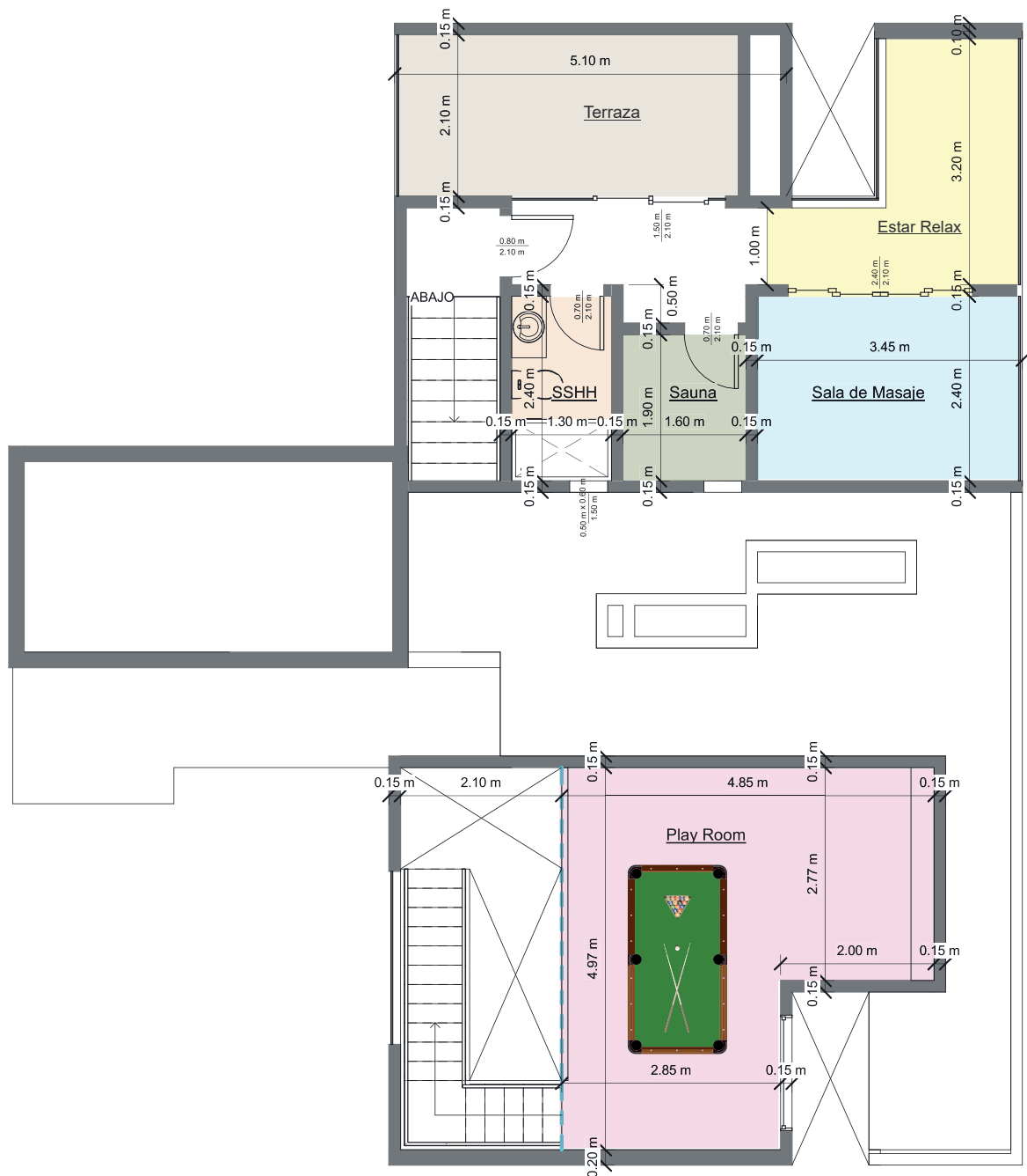
PLANTA TERRAZA 2
